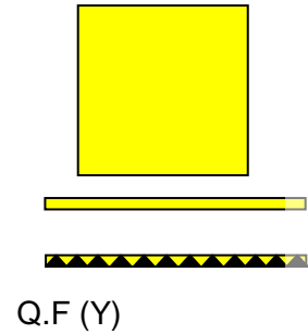
Hình 25: Báo hiệu đánh dấu khoang thông thuyền của công trình vượt sông trên không cho phương tiện cơ giới và thô sơ đi chung (B5.1)
